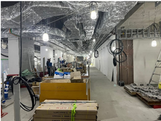
⑤地下駅舎部：プラットフォームの進捗状況 （建築・設備工事）※ホームドア工事着手前
