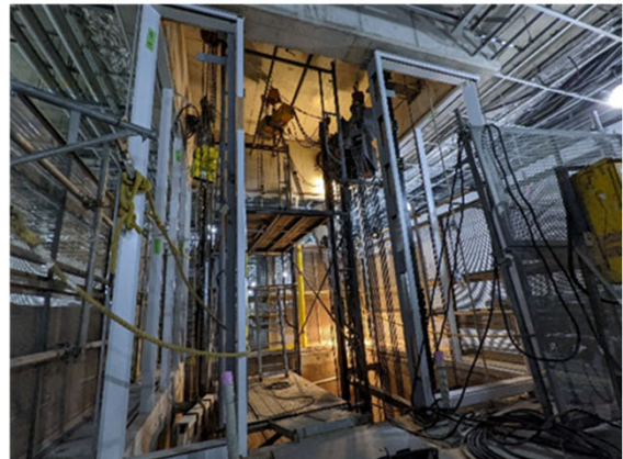
⑥地下駅舎部：プラットフォームの進捗状況 （ホームドア工事）
